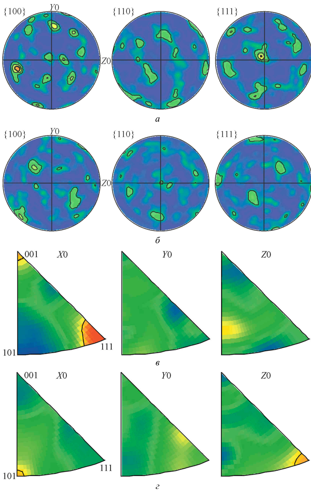
Рис. 5. Прямые ( a , b ) и обратные ( c , d ) полюсные фигуры рекристаллизованных зерен: a , c – исходные состояния; b , d – после ВЭ
